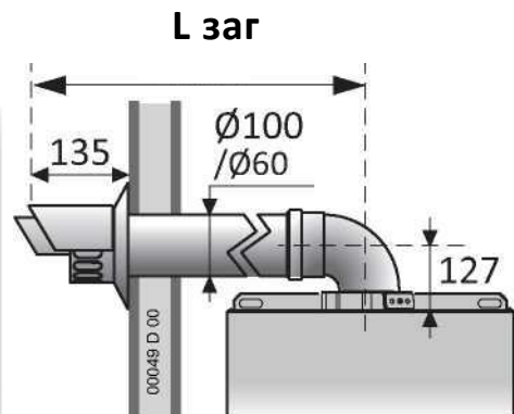
Приклад горизонтальної коаксіальної системи (C 13 )
